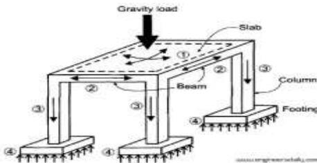
شكل (٤) يوضح مكونات الهياكل الخرسانية.
